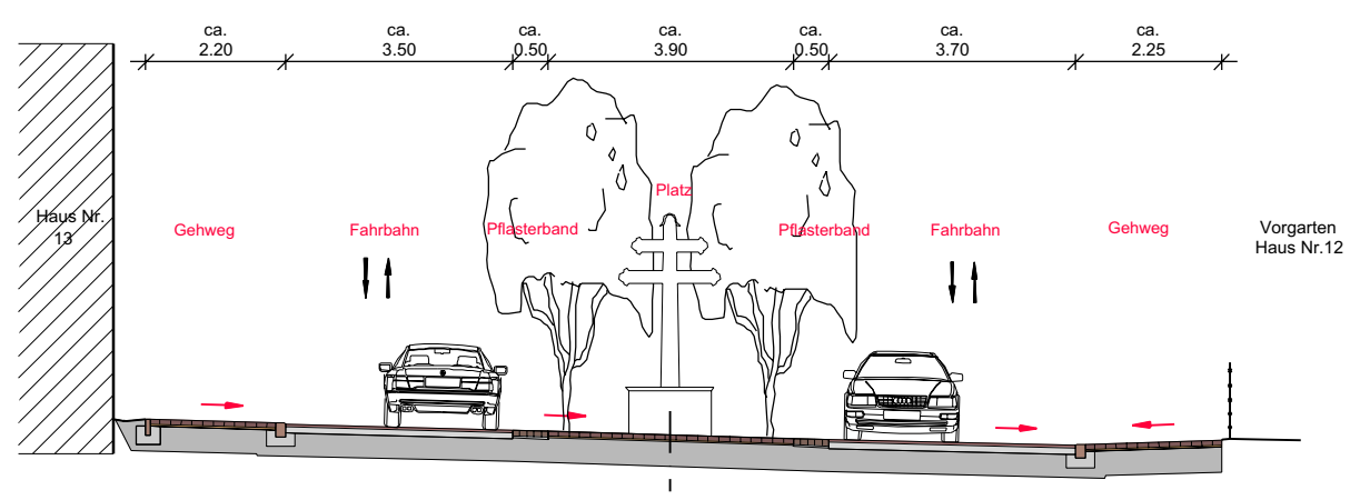
Regelquerschnitt I-I Umgestaltung Wilhelmsplatz, Hohenwart
